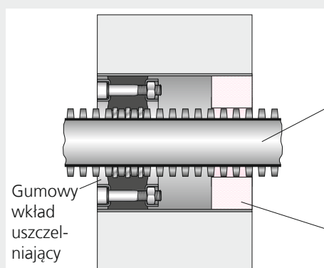
Przekrój zestawu uszczelniającego
